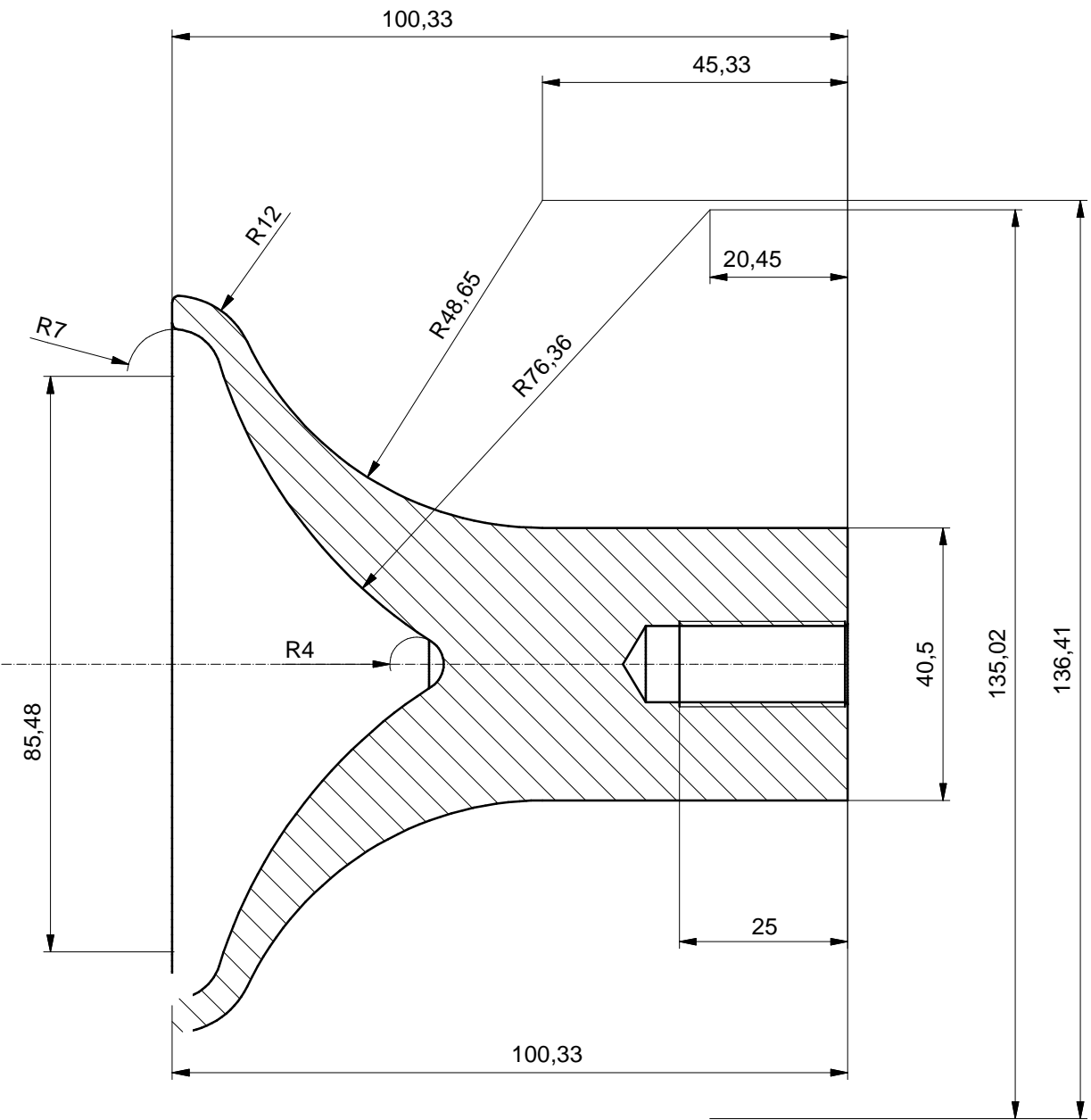
A-A (1:1)
